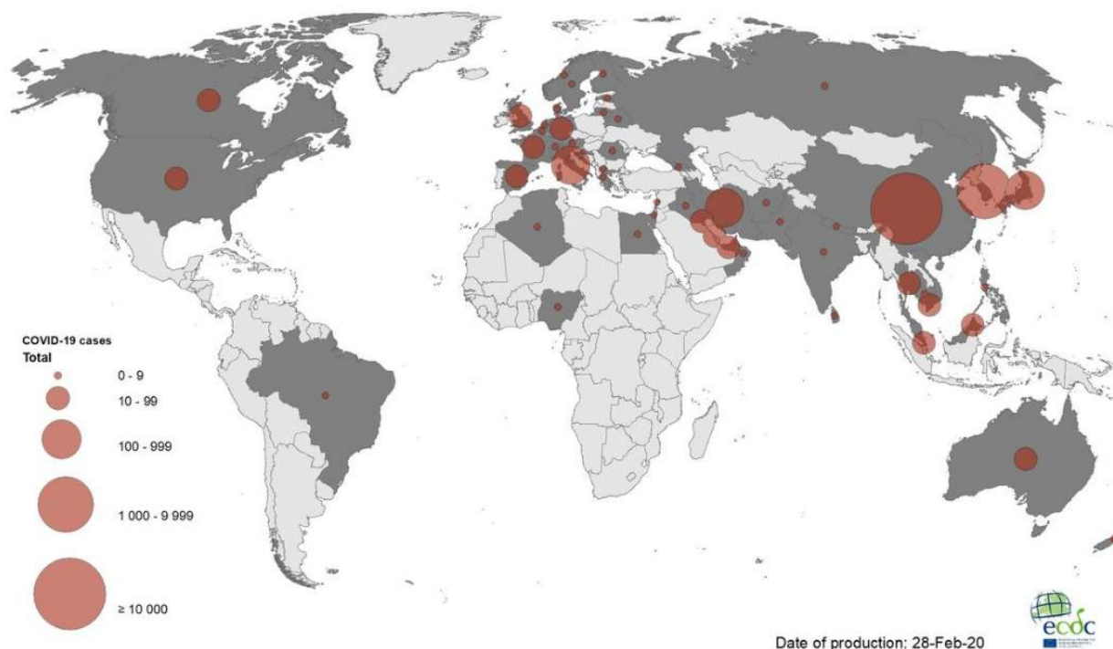
Figura 1. Distribuzione nel mondo dei casi di infezione da SARS-CoV-2 al 28-02-2020
